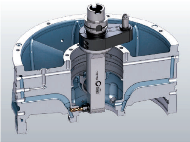
Cabeçote 90° longo
