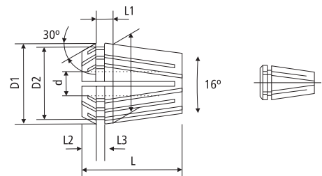
ER11 - ER50
